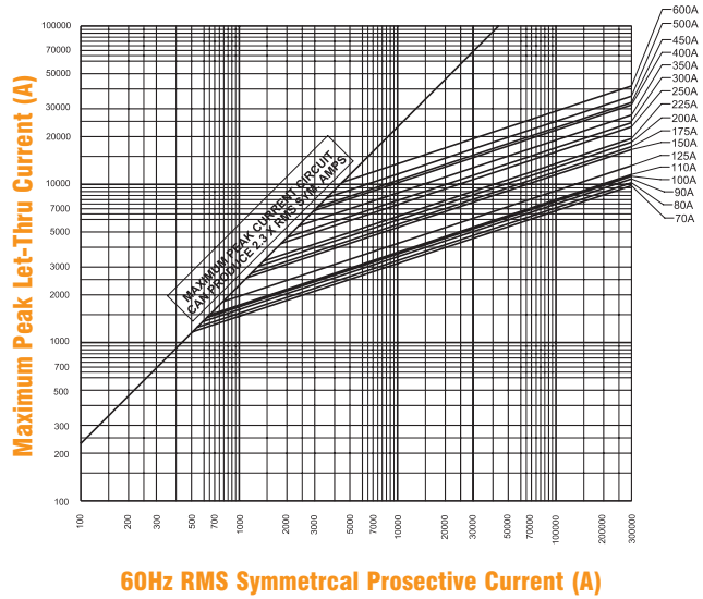
Peak Let-Thru Data HSRK70 — 600R, 600V AC
